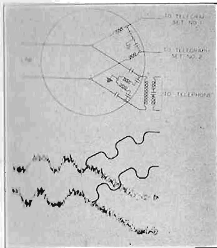
Fig. 4. Composite set.
