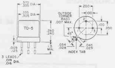
2N4037 2N3053
