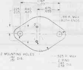
2N3055
