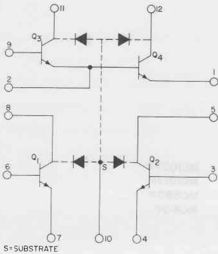
CA3018
