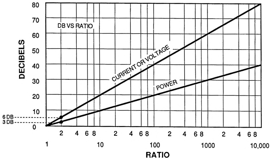
Decibels Vs Ratio
