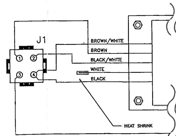
240 VOLT PRIMARY WIRING
