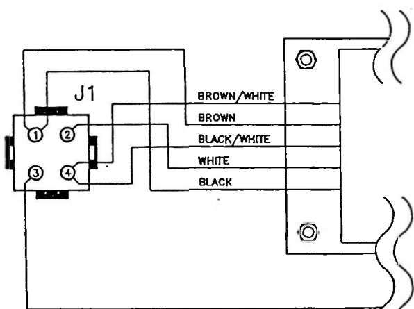
100 VOLT PRIMARY WIRING
