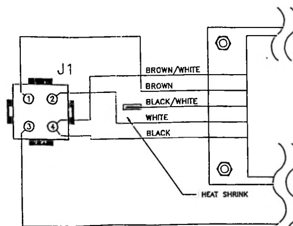
220 VOLT PRIMARY WIRING
