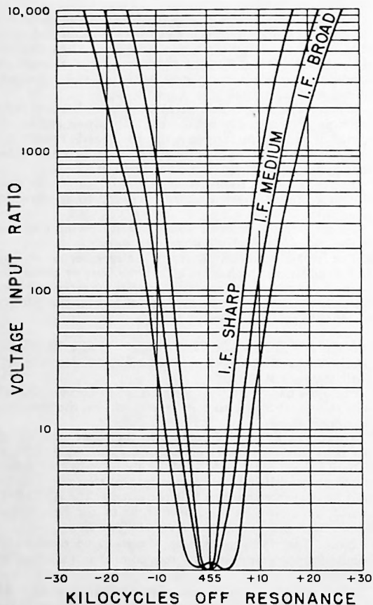
FIG. 1—I. F. SELECTIVITY
