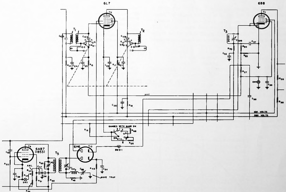
FIG. 5—NOISE LIMITER SCHEMATIC
