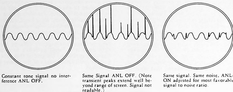
FIG. 6—NOISE LIMITER ACTION
