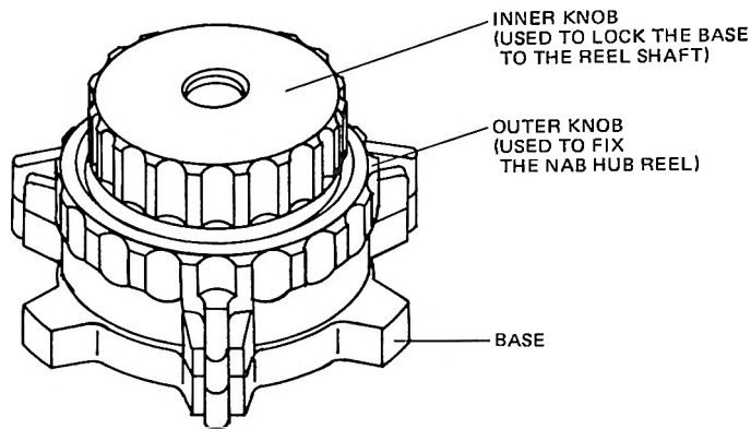
Fig. 3-1 Reel Hold Down Knobs
