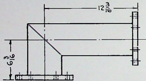
90° MITRE ELBOW MI-19314-C-18
