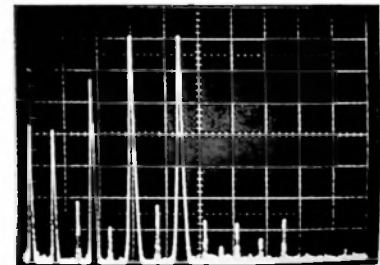
Fig. 62. 7 kHz L Minus R Im Test
