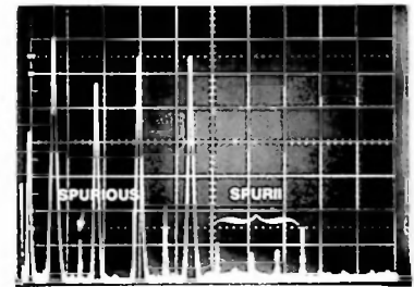
Fig. 61. 7 kHz Left Channel Im Test
